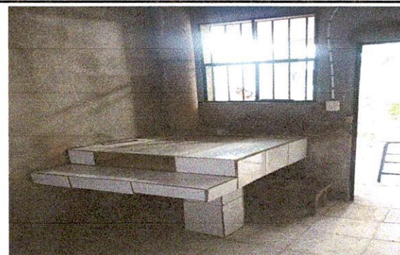
Foto 6: 19.2 SUSTITUCIÓN DE ESTUFA RURAL (COMPLETO) INCLUYE CHIMENEA Y PLANCHA DE METAL
