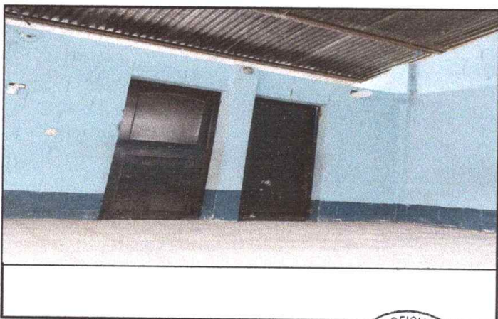
PUERTAS DE METAL: SUSTITUCION DE PUERTA (0.60M* 1.90M)
