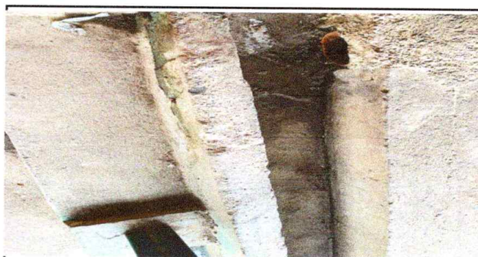
Foto 4: Reparación de bajada de agua pluvial, tubo PVC de 3"
