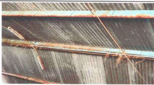
Foto No 2: Estructura de soporte de techo en mal estado.
