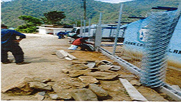
Foto1: reparacion de muro perimetral y maya calbanizada
