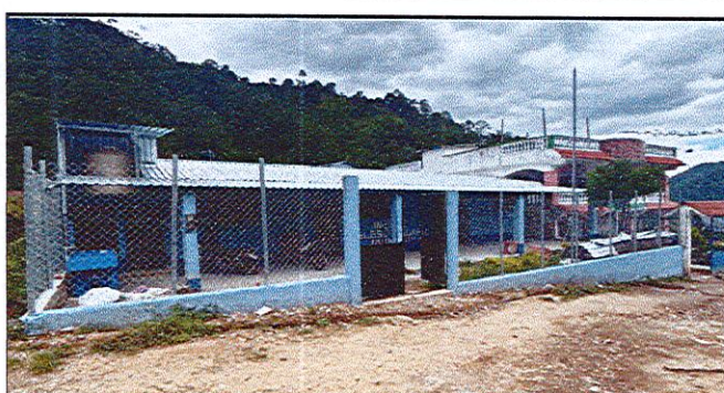
Foto 4: MURO PERIMETRAL CON MALLA Y TUBO GALVANIZADOS.
