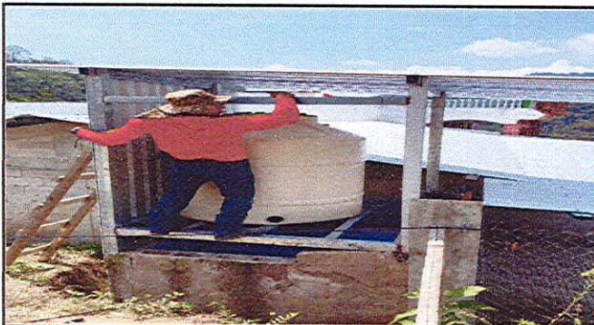
Foto 3: INSTALACIÓN DE DEPÓSITO DE AGUA 1,100 LITROS.
