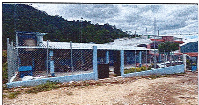
Foto 4: MURO PERIMETRAL CON MALLA Y TUBO GALVANIZADOS.
