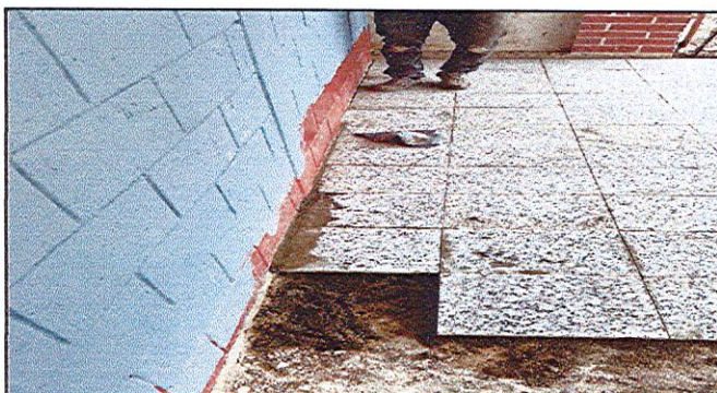
Foto 9: CAMBIO DE PISO, POR PISO DE GRANITO
