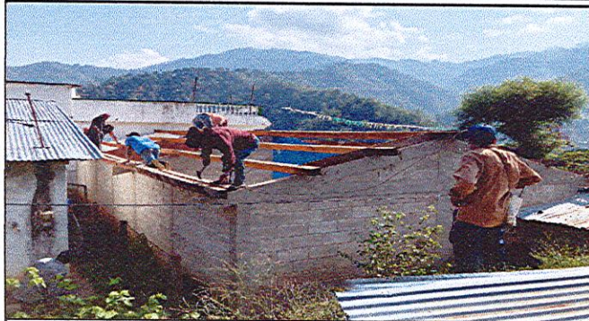
Foto 1: CAMBIO DE TECHO POR LAMINA TROQUELADA
