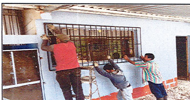
Foto 12: COLOCACIÓN DE BALCÓN DE METAL
