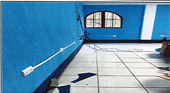
Foto7: Instalando tomacorrientes y cableado eléctrico para computadoras.
