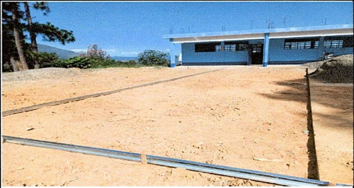
Foto. 8 Sustitución de piso de torta de concreto
