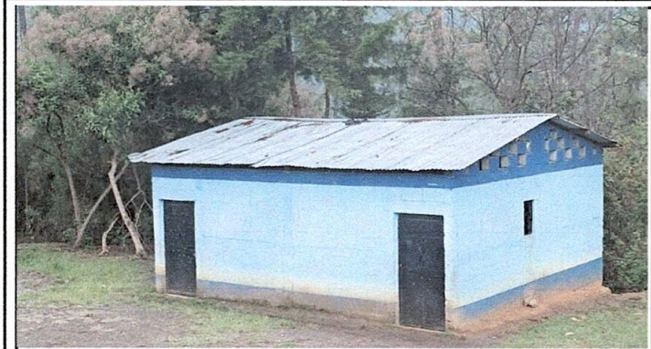
Foto1: Sustitución de lámina, por lámina troquelada aluzinc calibre 24
