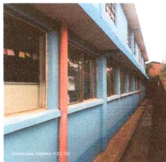
Foto 4: Sustitución de ventanas de aluminio por pvc más vidrio y mejoramiento de balcones de metal para aulas del primer piso del edificio escolar.
