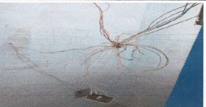
Foto 12: Cambio de cableado en lamparas de cancha polideportiva
