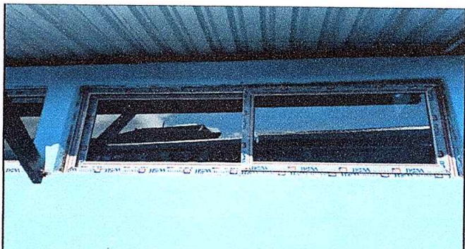
Foto 4: Colocación de ventanas corredizas para la cocina.
