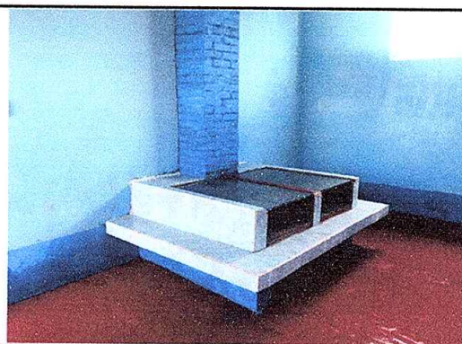
Foto 4: Sustitución de estufa rural (completa) incluye chimenea y plancha de metal
