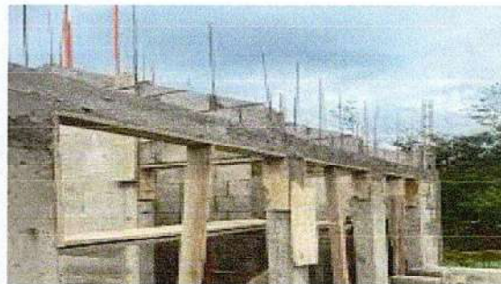
Foto 8: Estructura de techo: Colocación de estructura de soporte de metal.
