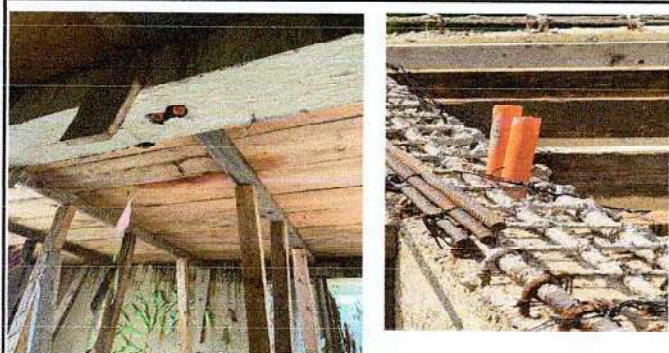
Foto1: Reparación del sistema eléctrico: Sustitución de sistema eléctrico (cable, focos, tomacorriente, plafoneras e interruptores)
