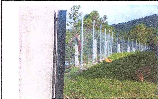
Foto 3: Reparación de tubo hg y malla galvanizada finalizada
