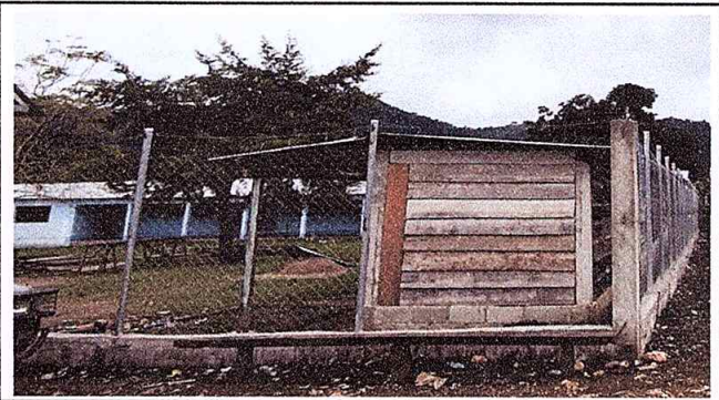
Foto 2: Muro perimetral con tubo HG y malla galvanizada ya terminado
