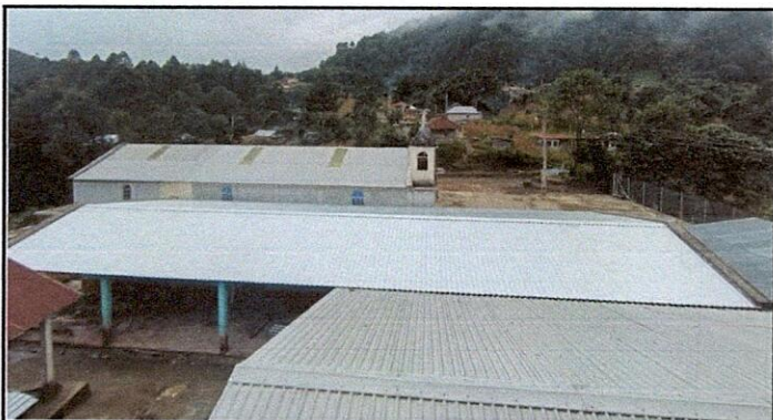
Foto 1.3: Sustitución de láminas, por láminas troqueladas
