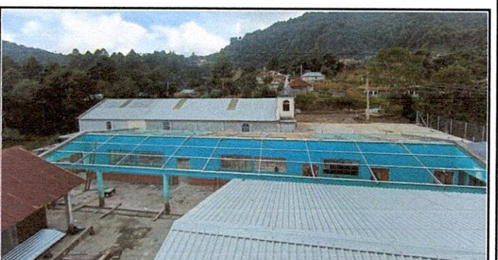
Foto 2.3: Sustitución de soporte de madera, por soporte de metal
