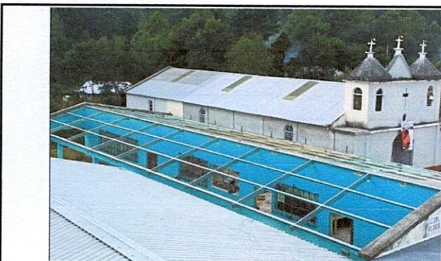
Foto 2.2: Sustitución de soporte de madera, por soporte de metal
