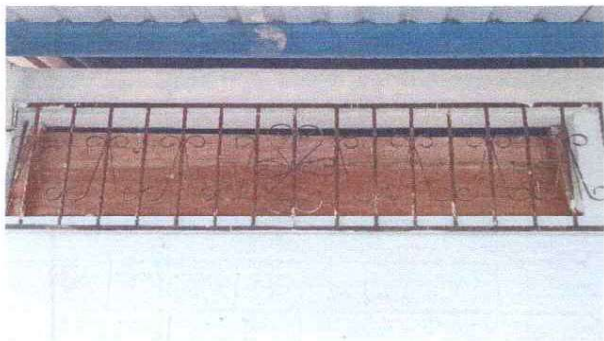
Foto 7: Sustitución de ventana de madera por metal mas vidrio 100 cms de altura X 200 cms de ancho
