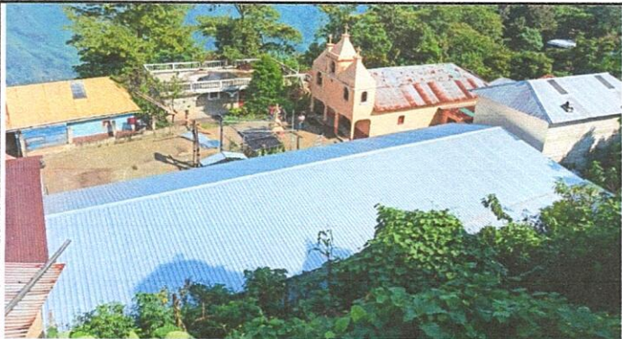
Foto 1.3: Sustitución de lámina, por lámina troquelada aluzinc calibre 26
