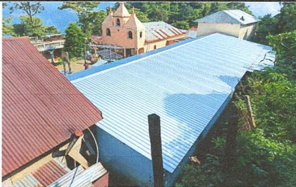
Foto 1.2: Sustitución de lámina, por lámina troquelada aluzinc calibre 26
