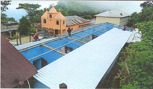
Foto1.1: Sustitución de lámina, por lámina troquelada aluzinc calibre 26
