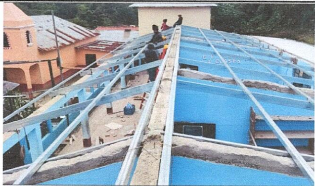
Foto 1.3: Sustitución de lámina, por lámina troquelada aluzinc calibre 26
