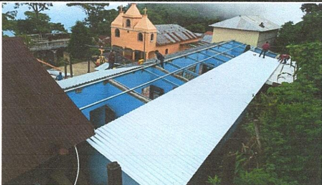
Foto 1.2: Sustitución de lámina, por lámina troquelada aluzinc calibre 26
