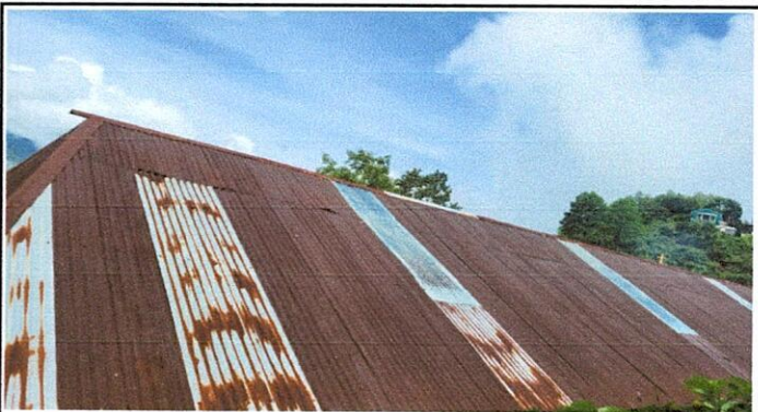
Foto 1.2: Sustitución de lámina, por lámina troquelada aluzinc calibre 26
