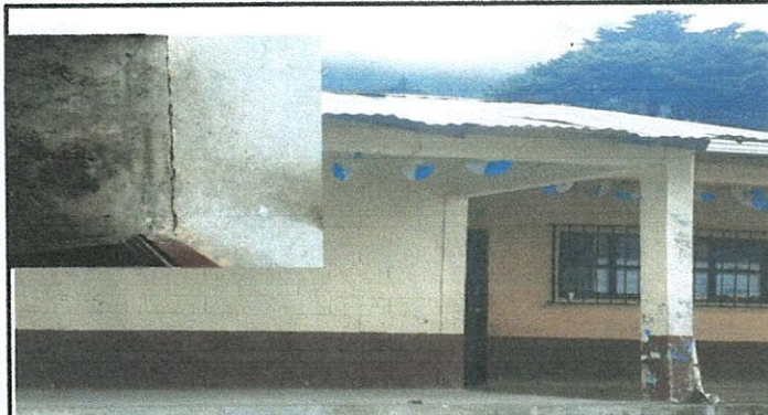
Foto 3: parte de en frente no cuenta con canal ni bajada de agua, afectando la pared por humedad.
