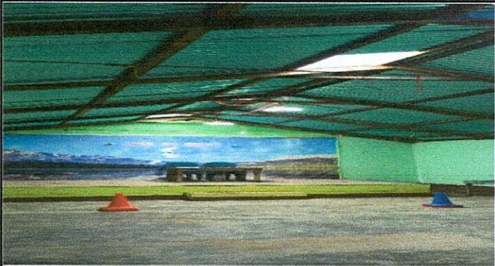
FOTO 3: Sustitución de estructura de soporte de madera por metal galvanizado
