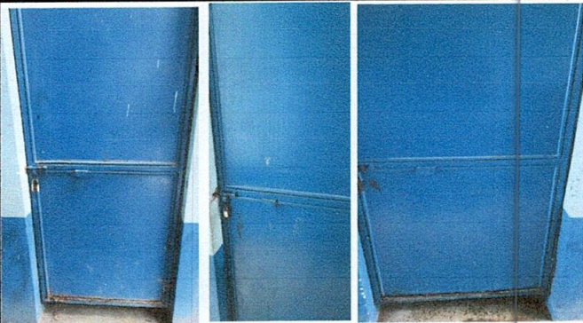
Foto 3: Sustitución de puerta de metal de 0.80 centímetros de ancho por 2.10 metros de alto
