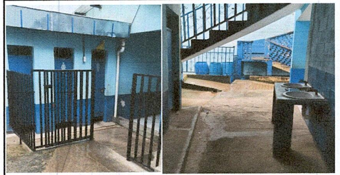
Foto 6: Sustitución de porton de metal de 1.89 metros de ancho por 2.10 metros de alto
