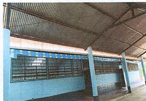
Foto 6: Sustitución de canal de metal
