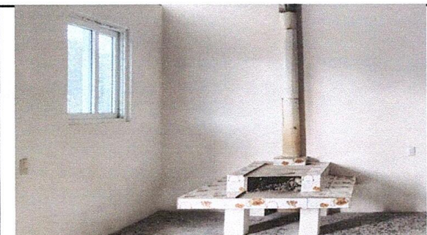
FOTO 3: Instalación de azulejo en estufa rural
