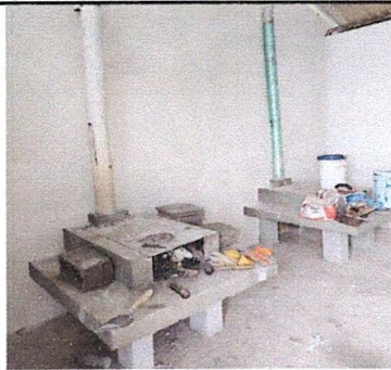
FOTO 3: Instalación de azulejo en estufa rural
