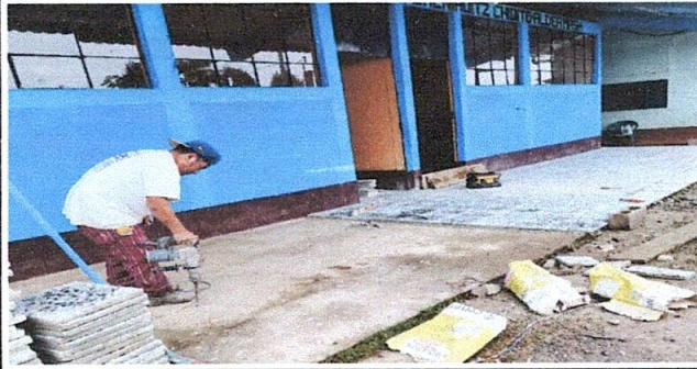
FOTO 7: Sustrucción de piso de granito
