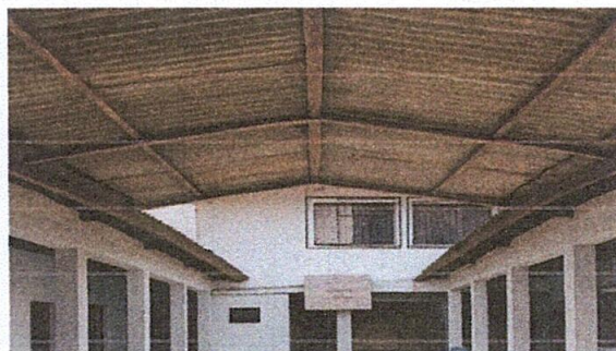
Foto 2: ESTRUCTURA DE TECHO Y CUBIERTA DE LAMINA
