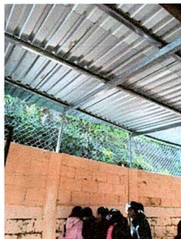
Foto 2: Sustrucción de lámina, por lámina troquelada aluzinc calibre 26
