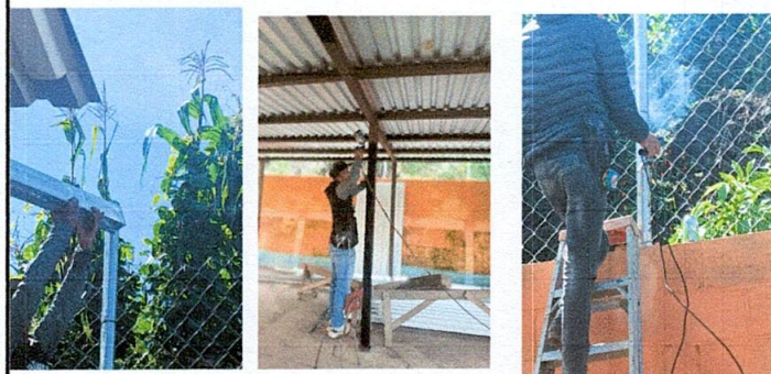
Foto1: Sustitución de estructura de soporte de madera por metal
