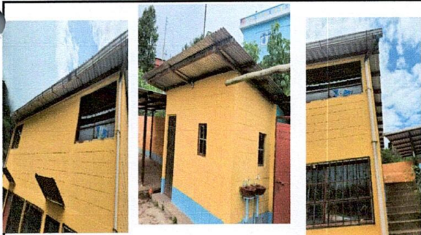
Foto 11 Sustrución de canales de metal y bajadas de agua pluvial tubería PVC 3"
