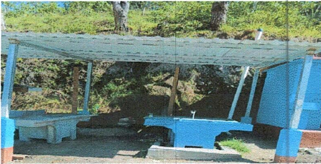
Foto 1: Sustrucción de estructura de soporte de madera por metal y Sustrucción de lámina, por lámina troquelada aluzinc calibre 26
