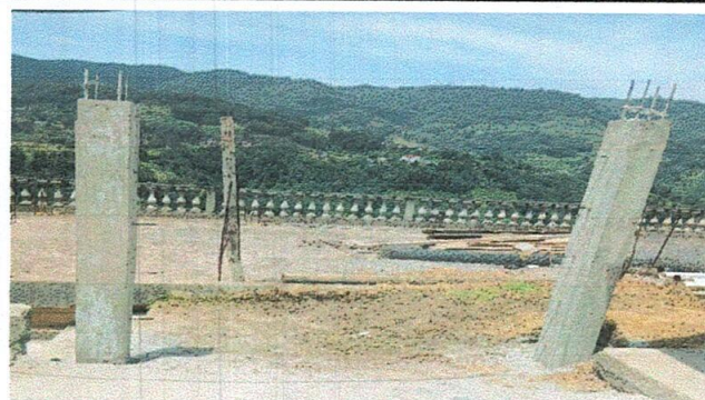
Foto 2: Mejoramiento de porton de metal de 5.50 metros de ancho por 2 metros de alto
