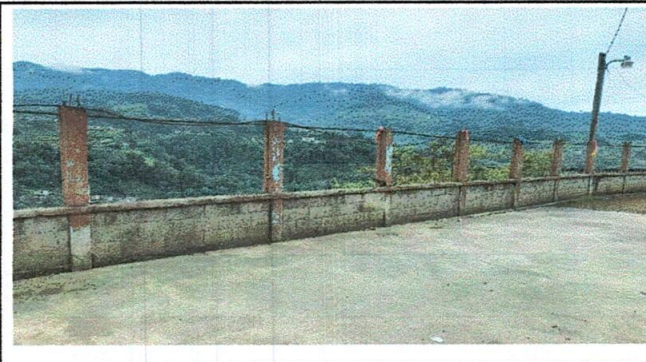
Foto 6: Sustitución de tubo hg y malla galvanizada
