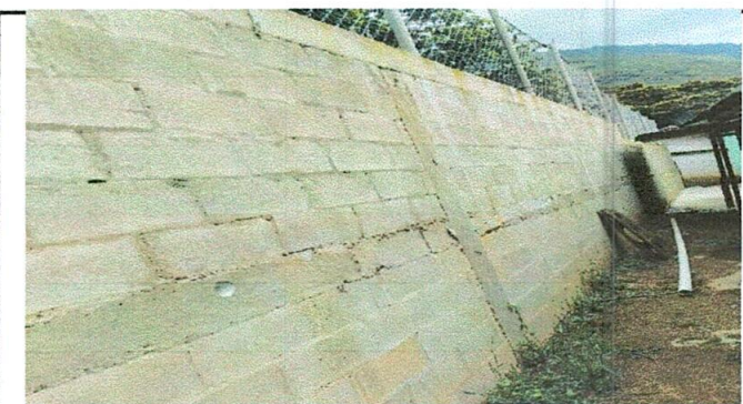
Foto 5: Mejoramiento de pepello en muro
