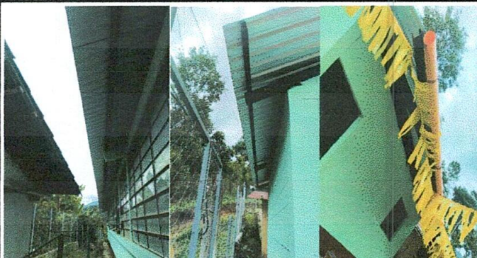
Foto 3: Mejoramiento de canal de metal y Mejoramiento de bajada de agua pluvial tubo PVC 3"
