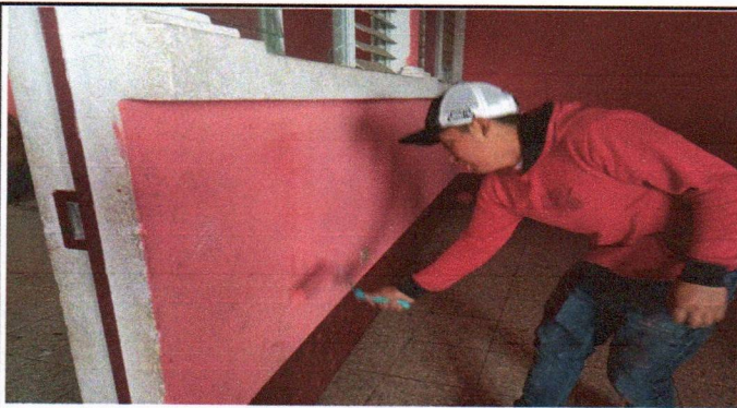
Foto9: Aplicando pintura de exteriores aula cuatro.
