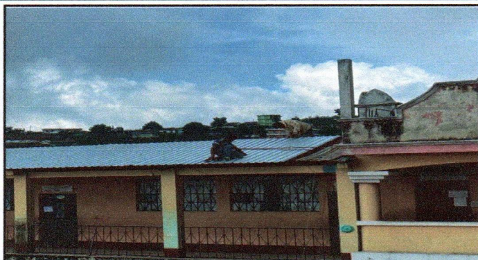
Foto1: colocacion de lámina troquelada calibre 26
