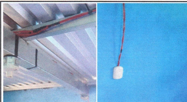
Foto 8: Sustitución de cableado electrico
