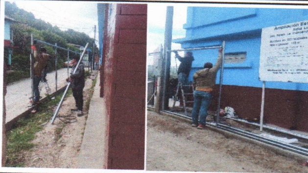
Foto 7: Reparación de tubo hg y malla galvanizada
