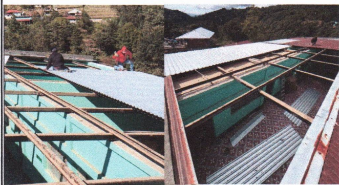
Foto1: Sustitución de láminas por lamina troquelada
