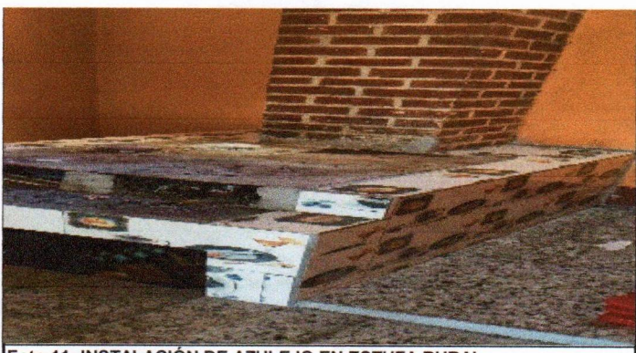
Foto 11: INSTALACIÓN DE AZULEJO EN ESTUFA RURAL
