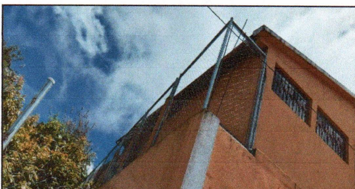
Foto 18: SUSTITUCIÓN DE ELEMENTOS DE FIJACIÓN, HIERROS PLANAS DE 3/4
