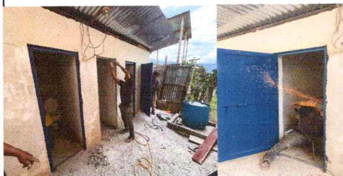
Foto 3: así se está trabajando la sustitución de 4 puertas en mal estado de servicios sanitarios de 160 cms de altura y 60 cms de ancho.
