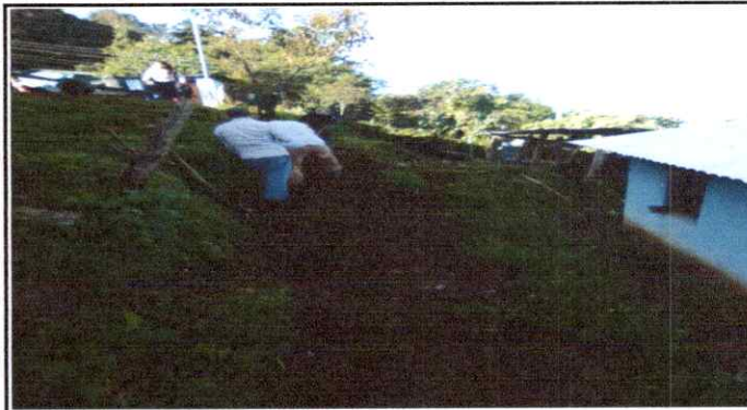
Foto 14: Sustitución de tubería PVC línea principal aguas negras
