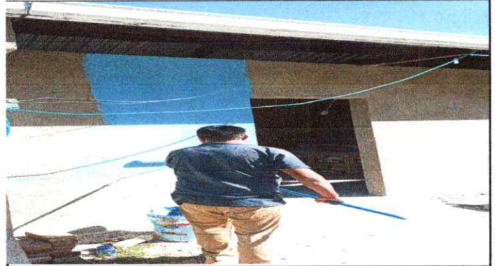
Foto 8: Pintura en muros exteriores e interiores
