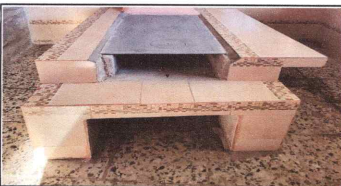
Foto 23: Instalación de azulejo en estufa rural
