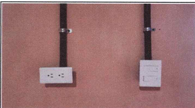
Foto 21: Instalación unidad de fuerza (tomacorrientes, flipones y tableros)
