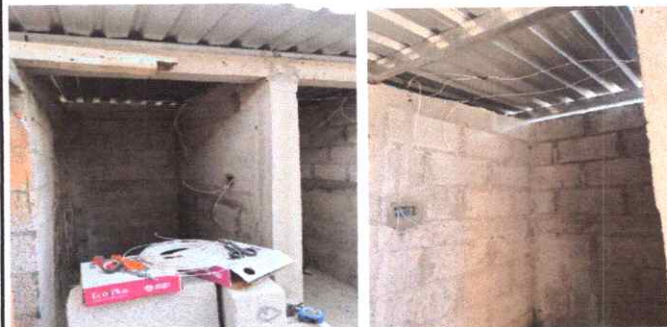
Foto 2: 10.1, 10.2, 10.3, 10.4 Sustitución de: cableado eléctrico, plafoneras, interruptores y focos ahorradores
