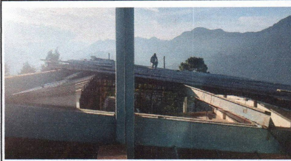
FOTO No. 2 INICIO DE LA VAJA DEL TECHOS DEL SALON
